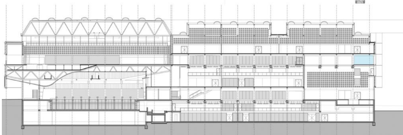
sección | secció | section
